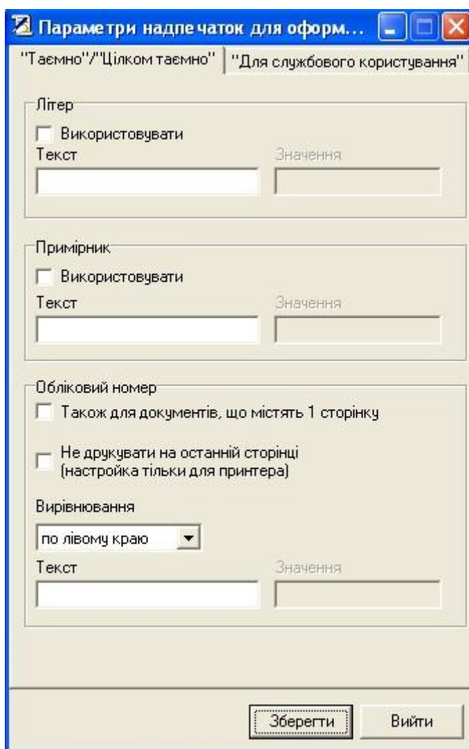
Рисунок 3.15 –Шаблони для оформлення документів
